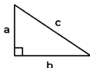
شکل (۹). قضیه منسوب به فیثاغورس در محاسبه وتر مثلث قائم‌الزاویه
