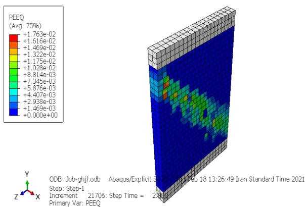
شکل ۷. توزیع کرنش پلاستیک معادل (PEEQ) در دیوار بنایی بدون تقویت تحت بارگذاری چرخه‌ای
