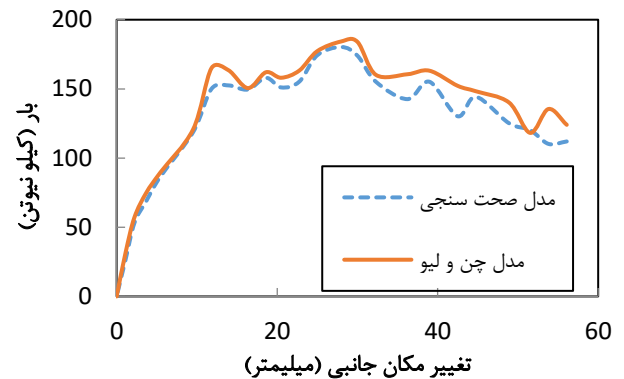
شکل ۵. مقایسه منحنی نیرو-تغییر مکان بین مدل عددی حاضر و نتایج آزمایشگاهی چن و لیو [۱۴]
