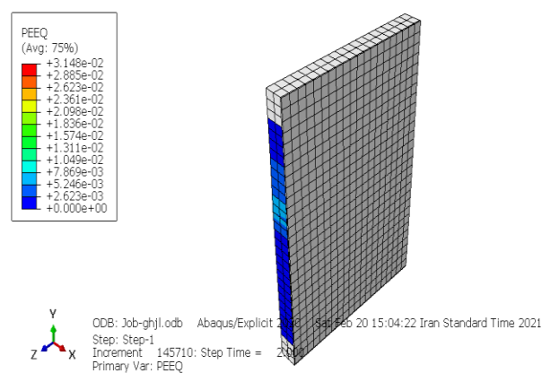
شکل ۸. توزیع کرنش پلاستیک معادل (PEEQ) در دیوار بنایی تقویت شده با الیاف شیشه تحت بارگذاری چرخه‌ای
